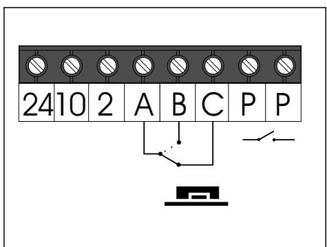
10. Aansluiten deuropener.
